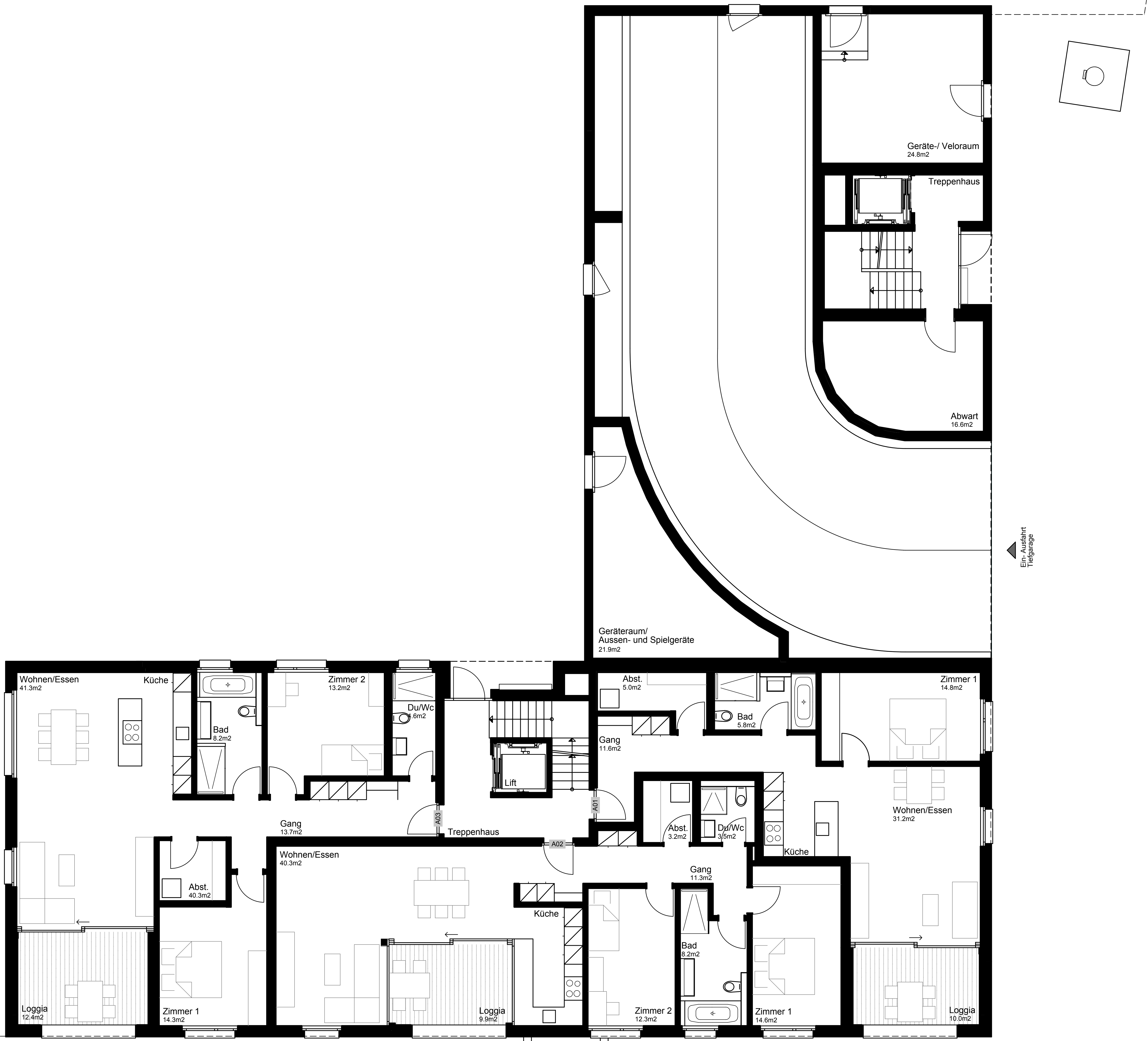
Wohnung A03 3¼ Zi- Whg. Wohnfläche: 105m 2
