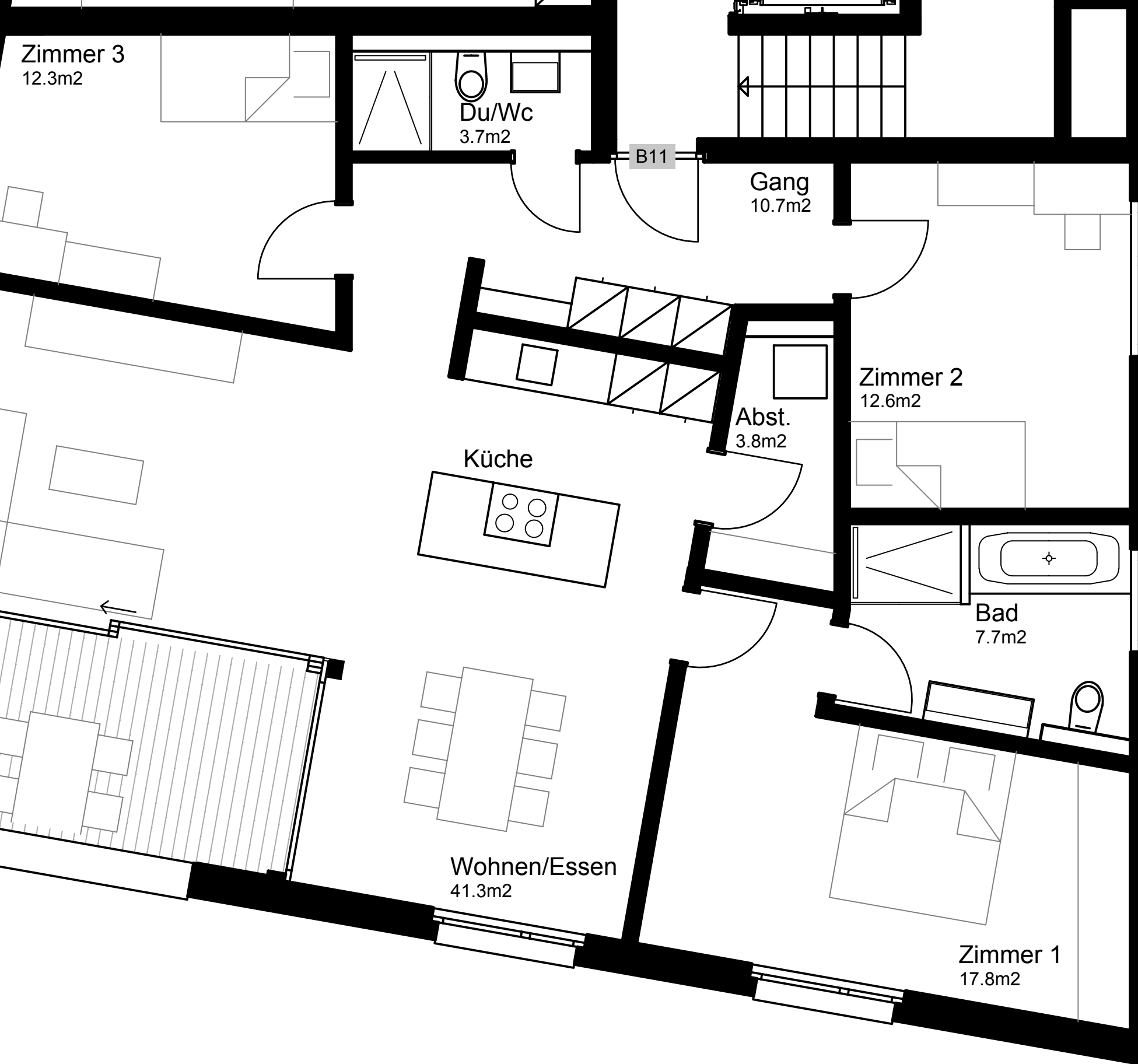
Wohnung B11 4½ Zi- Whg. Geschossfläche: 116m²
