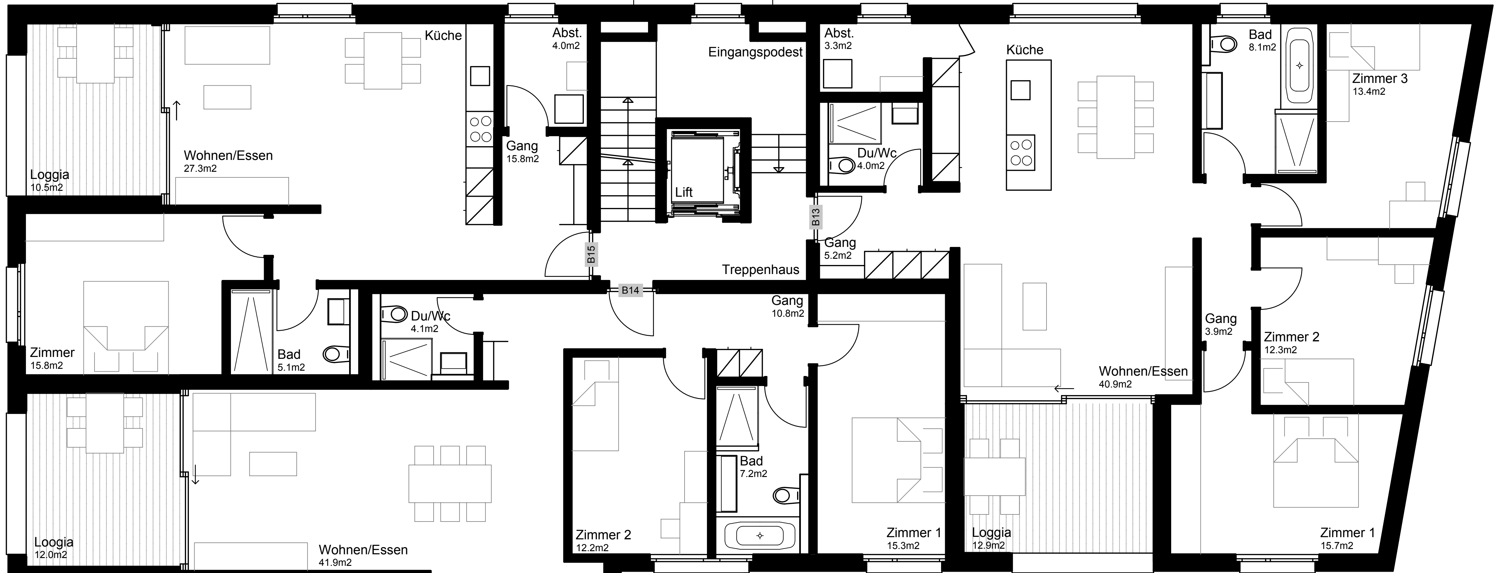
Wohnung B13 4½ Zi- Whg. Geschossfläche: 113m²
